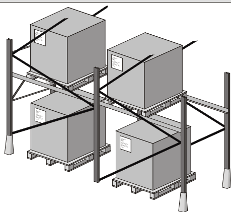
ГЛУБОКИЙ СТЕЛЛАЖ
